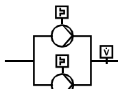
Управление сдвоенным насосом с наблюдением за протоком и перегрузкой
