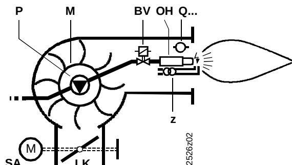
Принцип работы горелки с принудительной тягой
