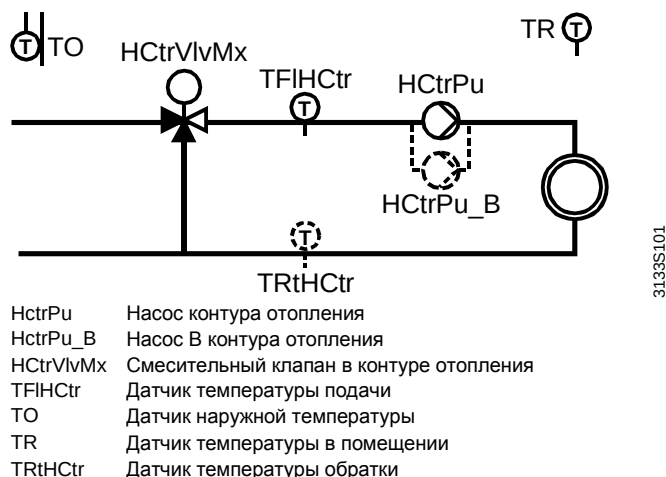
Схема контура отопления
